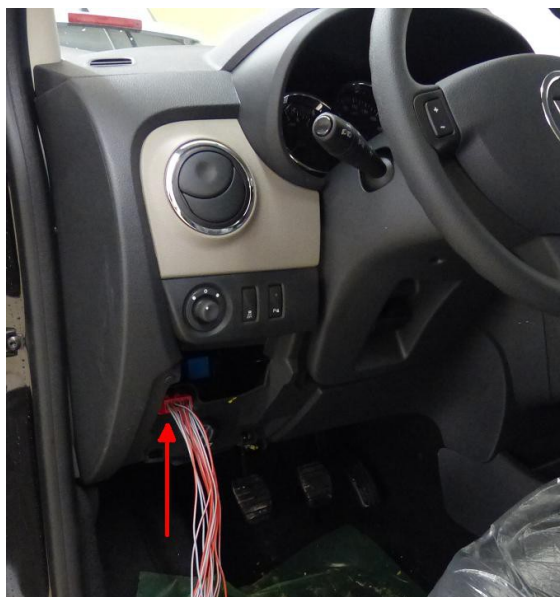
Abbildung 1: OBD Buchse
